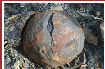
Kalkbolle
